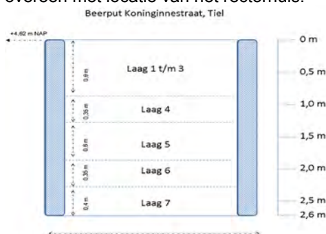
Afbeelding 14: Tekening van de beerput met hierin de hoogte van de aangetroffen lagen. Vermeldenswaardig is dat de NAP hoogte van de top van de beerput significant afwijkt 52 t.o.v. de gepubliceerde ROB resultaten.
